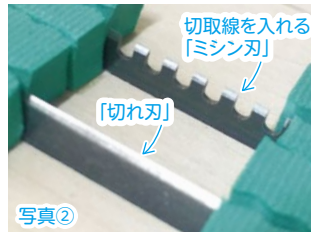
▲刃の拡大写真です。「切れ刃」(写真②)は化粧箱展開図の外形などを切ります。折り目を入れるための「スジ刃」(写真③)は刃先が丸く、「切れ刃」よりも高さが低くなっています。
