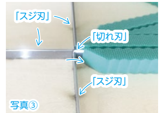
▲刃の拡大写真です。「切れ刃」(写真②)は化粧箱展開図の外形などを切ります。折り目を入れるための「スジ刃」(写真③)は刃先が丸く、「切れ刃」よりも高さが低くなっています。
